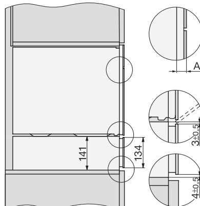
Seitenansicht_DG_DGM_ESW7x10_EVS7010, Skizze
